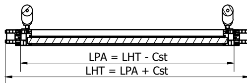
A-A ( 1:10 )
